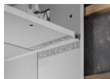
Kit profil de construction (2m) pour le crépissage (montage en coin) SMALL CORNER DC 38/36 gris avec couvercle blanc dépoli FXZA4573 (2m)
