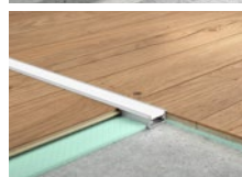
Kit de profils de sol avec ailes (1m/2m) plat SMALL W FLOOR 27/11 gris Avec couvercle blanc dépoli Résistant jusqu'à 500 kg FXZA4568 (1m) FXZA4569 (2m)
