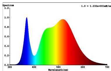
LED-Retrofit-Reflektorlampen 4000K
