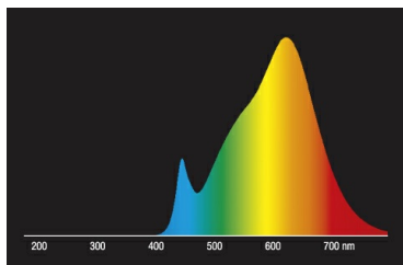
LED-Retrofit-Reflektorlampen AR111 827
