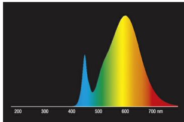
LED-Retrofit-Retrofitlamps 3000K
