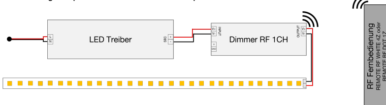
Verdrahtungsbeispiel für einfache weiße LED Strips
