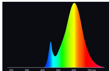
RaLEDina: LED retrofit pour tubes à incandescence 2700K
