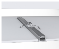
Clip de montage pour profil S, Bracket spring SMALL B1
