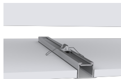
Clip de montage pour profil M, Bracket spring MEDIUM B2
