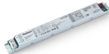
Driver DALI pour lampes et modules LED DC, 60W/1100-1500mA IP20
