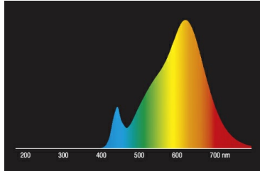
LED-Retrofit-Reflektorlampe MR16 / PAR16 2700K
