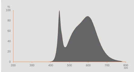
LED-Retrofit-Reflektorlampen 4000K
