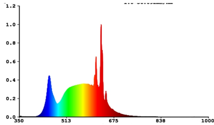
LED-Retrofit-Lampen 4000K, sehr gute Farbwiedergabe Ra 90
