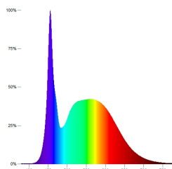
LED-NEO-Tubes 6500K, Remplacements pour lampes fluorescentes
