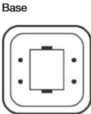
G24q IEC/EN 60061-1 sheet 7004-78-5
