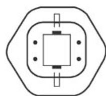
GX24q IEC/EN 60061-1 sheet 7004-78-5
