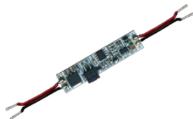
Einbau-Sensor für Aluprofile, In-Profile DOOR Sensor 96W/12-24V
