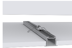
Montageclip für Profil M, Bracket spring MEDIUM B2
