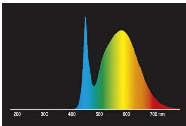
LED-Retrofit-Reflektorlampen 4000K
