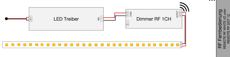
Verdrahtungsbeispiel für einfache weiße LED Strips
