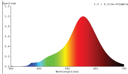
LED-Strip WarmDim @2700K, Ra min. 90
