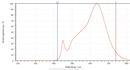
LED-Strip TW, Referenzfarbtemperatur 2700K, Ra 80
