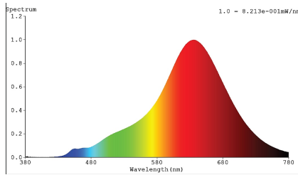
LED-Strip WarmDim @2700K, Ra min. 90
