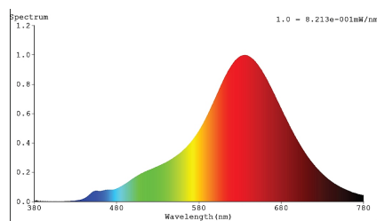
LED-Strip WarmDim @2700K, CRI min. 90
