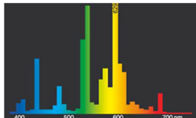
Teinte de lumière 827 Spectralux® Intra (41)
