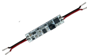
Einbau-Sensor für Aluprofile, In-Profile WINK Sensor 96W/12-24V
