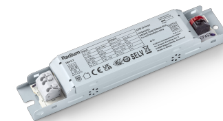
Driver pour lampes et modules LED DC, DRIVER 15W/350mA IP20
