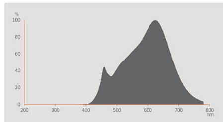
LED-Retrofit-Retrofitlampen 3000K
