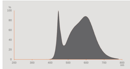
LED-Retrofit-Reflektorlampe 4000K
