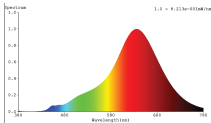
LED-Strip WarmDim @2700K, Ra min. 90
