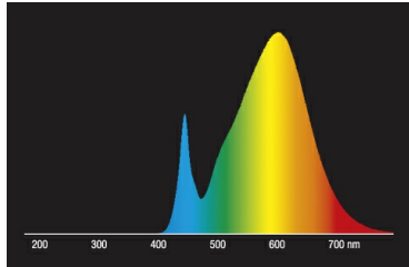
LED-Retrofit-Standardlampe 40W Ersatz, 2700K
