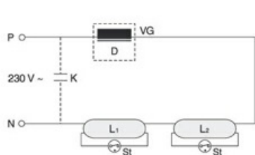
Tandem- oder Reihenschaltung mit VVG
