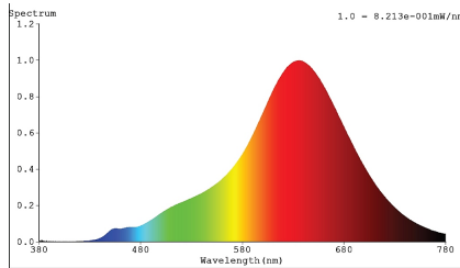
LED-Strip WarmDim @2700K, CRI min. 90
