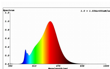
LED-Strip 2700K, Ra min. 90
