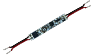
Einbau-Sensor für Aluprofile, In-Profile TOUCHDIM Sensor 72W/12-24V
