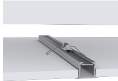
Embout pour profil et couvercle M, Endcap MEDIUM Profil d'angle 52/9.5
