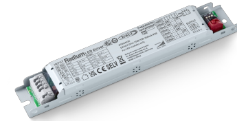
Driver DALI pour lampes et modules LED DC, 15W/100- 350mA IP20
